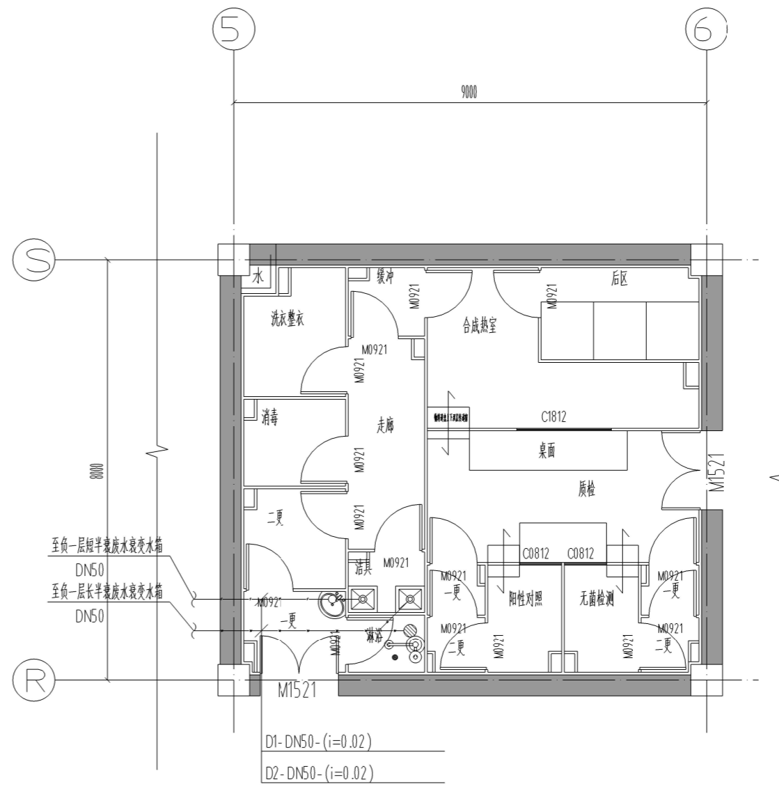
一层排水平面图
