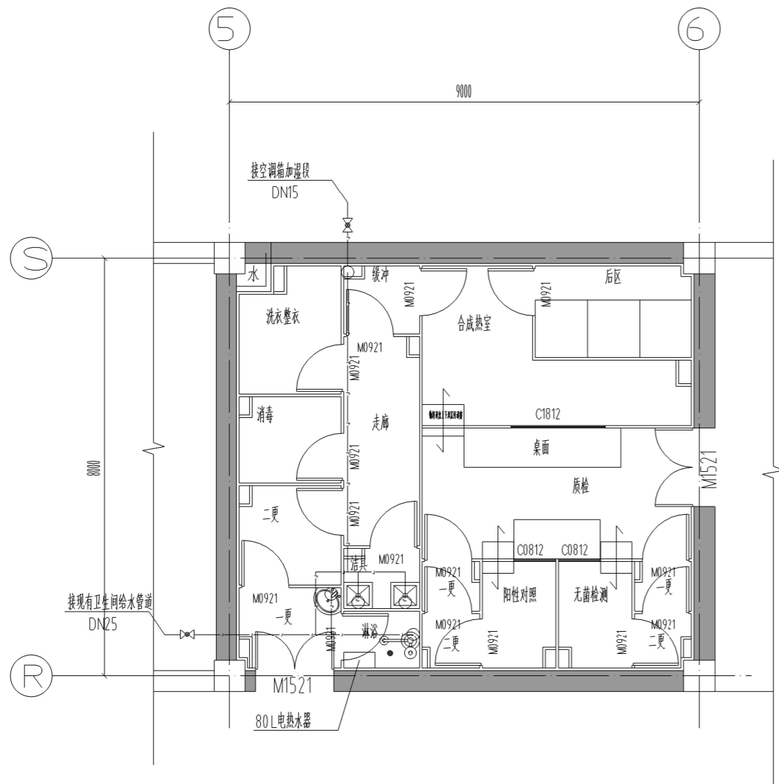
一层给水平面图
