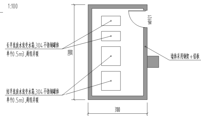
衰变水箱平面图
