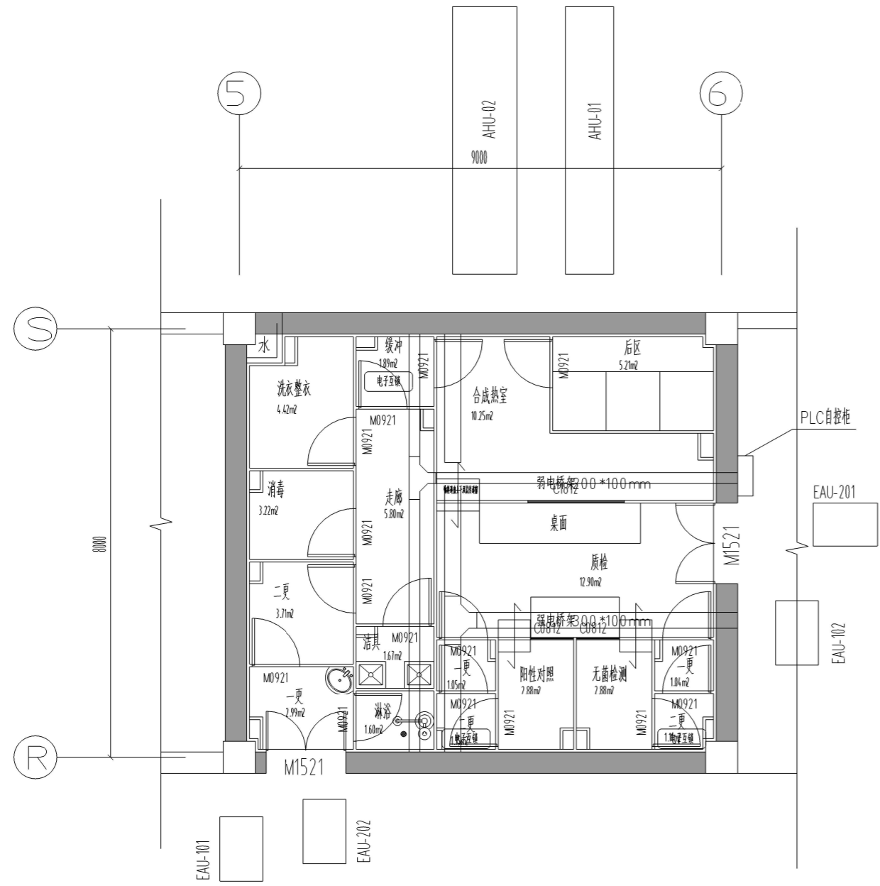
一层自控平面图 1:100
