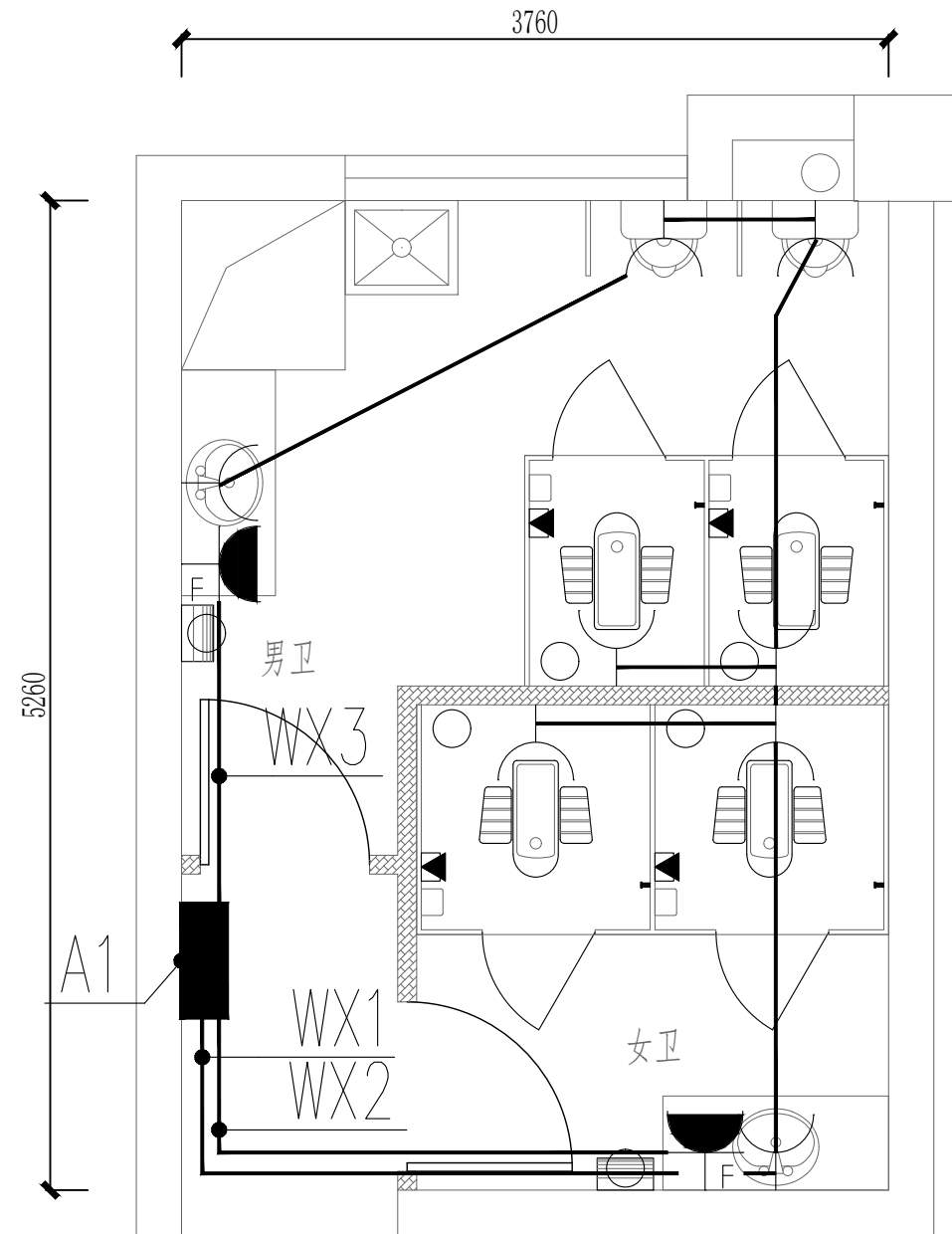
5、7、8F 中卫生间配电平面图
