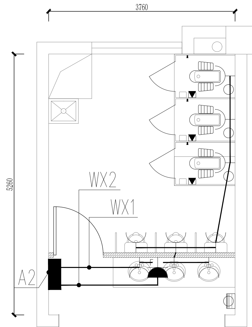
3、4、6F 男西卫生间配电平面图
