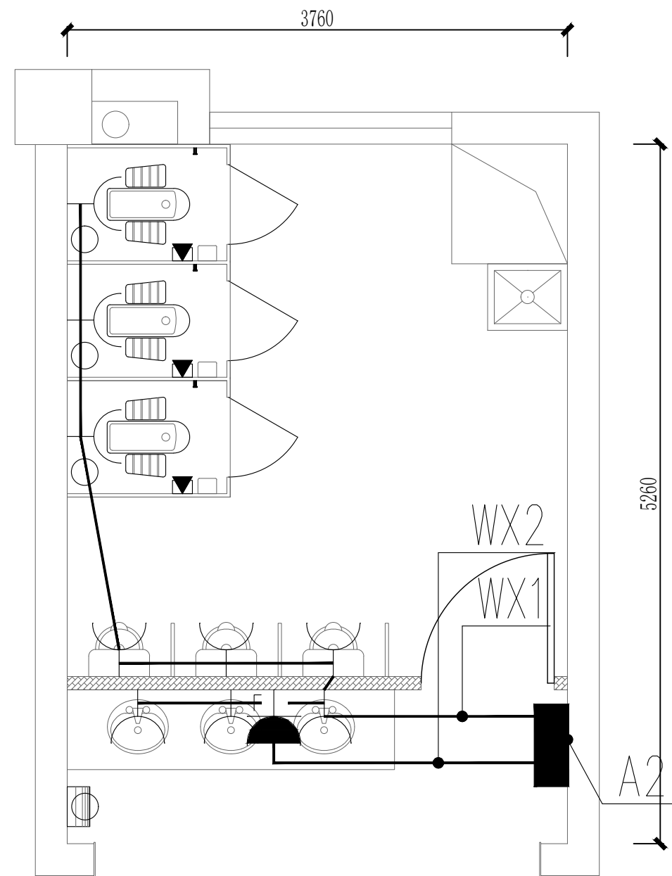
3、4、6F 男东卫生间配电平面图
