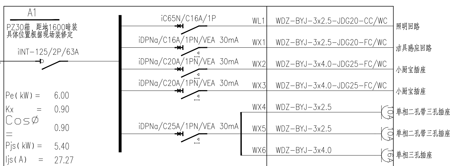
A1 配电箱系统图
