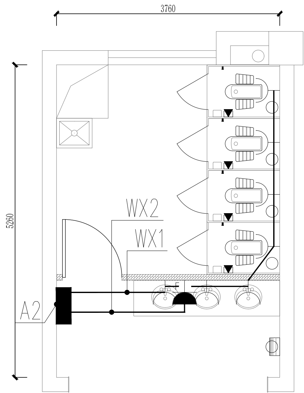
3、4、6F 女中卫生间配电平面图
