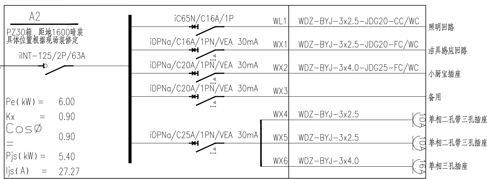
A2 配电箱系统图
