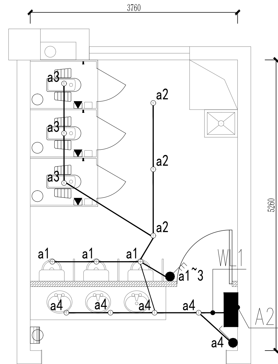
3、4、6F 男东卫生间照明平面图
