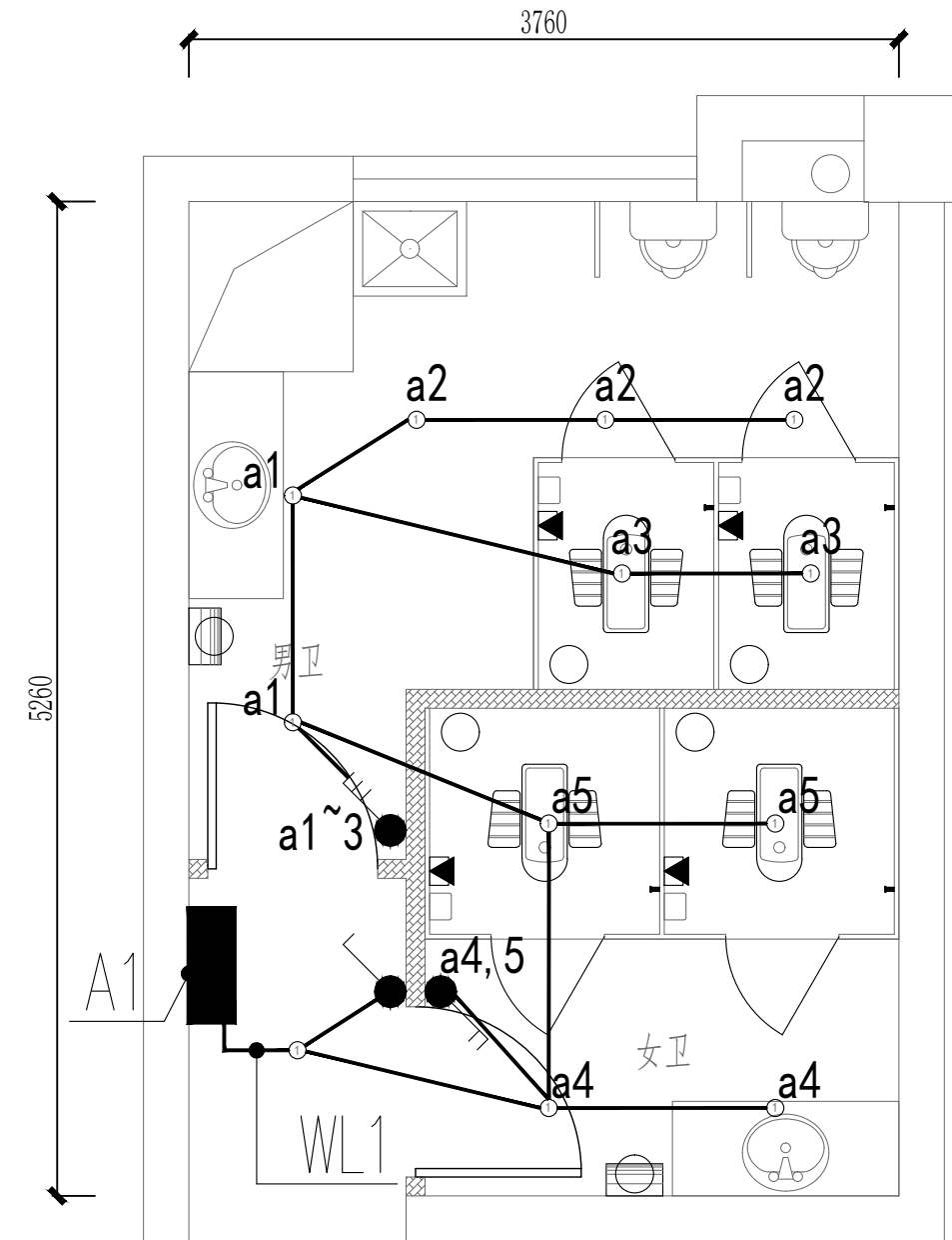
5、7、8F 中卫生间照明平面图
