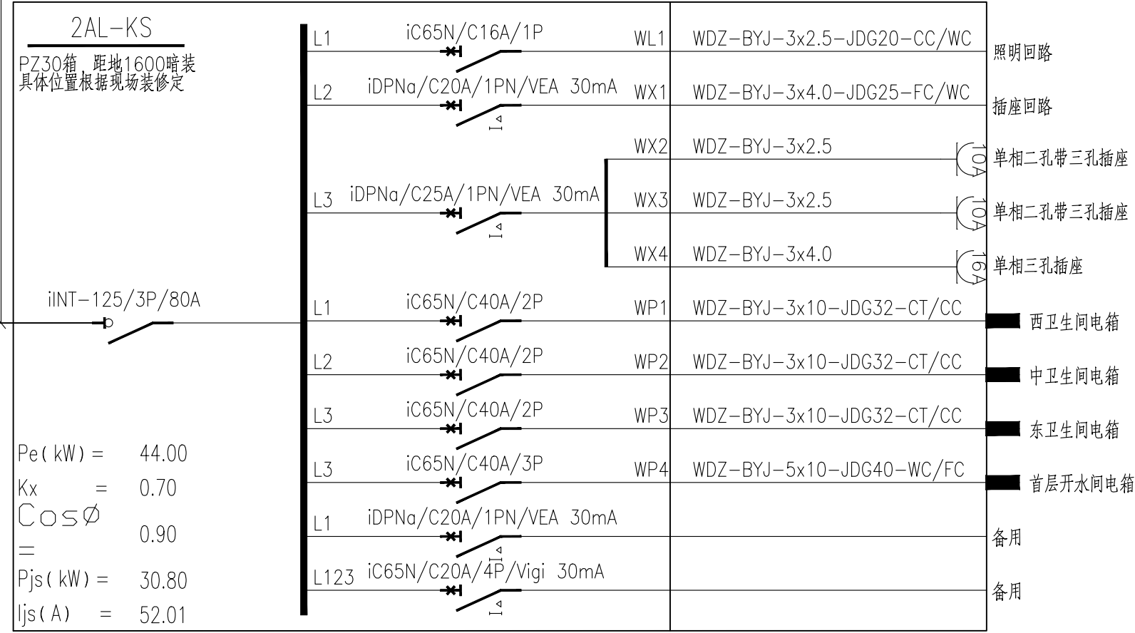
2F 开水间配电箱系统图
