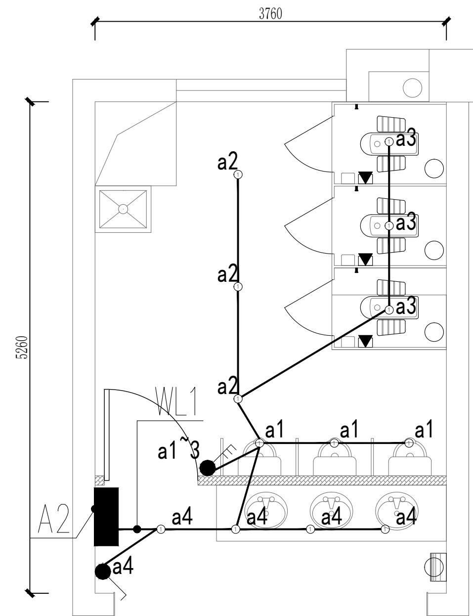
3、4、6F 男西卫生间照明平面图
