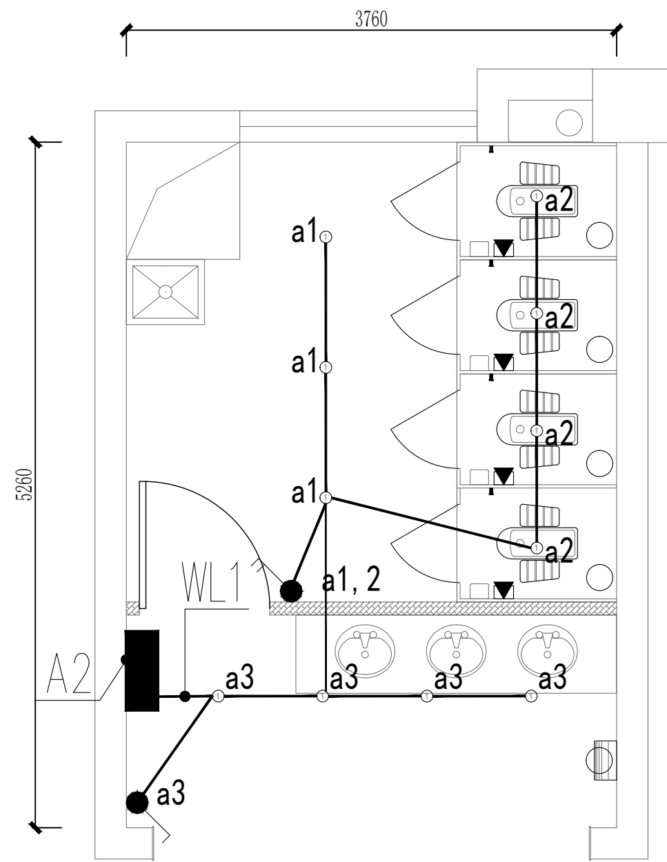
3、4、6F 女中卫生间照明平面图
