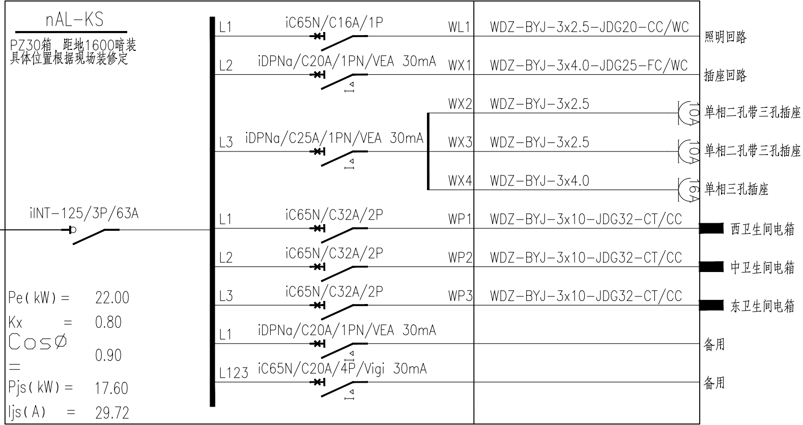
开水间配电箱系统图
